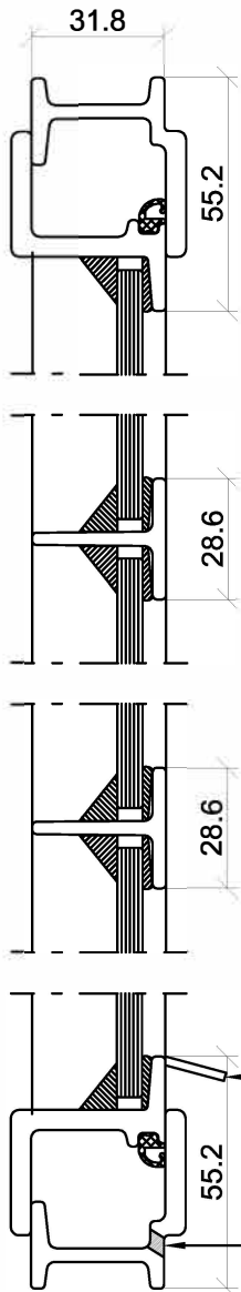
1 Scale: 1:2
